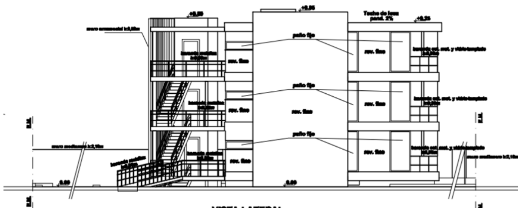
VISTA LATERAL S/ CALLE LOS BAQUEANOS Esc. 1:100
