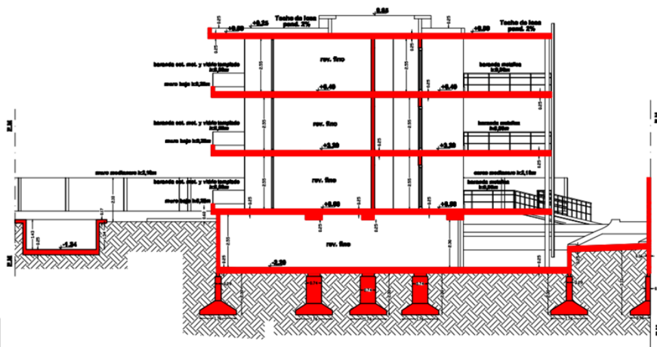
Corte B-B
